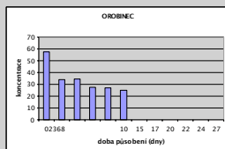
Obr. 4. Odbourávání pentritu. Odpadní voda z výroby pentritu (pentaerythritetrahydrátu, PETN) obsahovala pentritu více než 60 mg.dm -3 , v modelových čistírnách byl pentrit z odpadní vody odbourán po 10 dnech v případě kontejnerů osázených sítinou a orobincem, v případě rákosové kultury došlo k odbourání pentritu pod detekční limit po 15 dnech.
